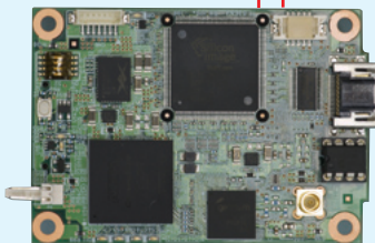
HDMI I/Fボード
